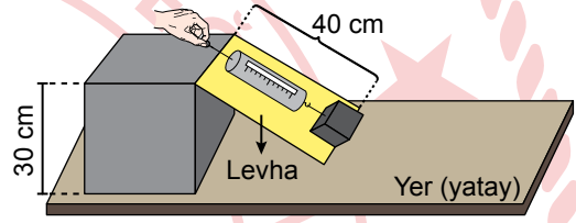
II. Düzenek
